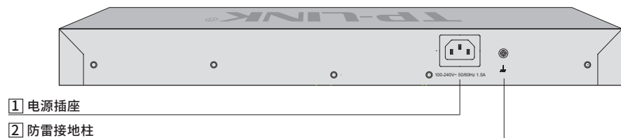
图1-2 TL-SH6428F后面板示意图
