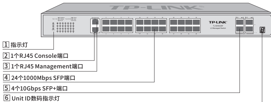
图1-1 TL-SH6428F前面板示意图
